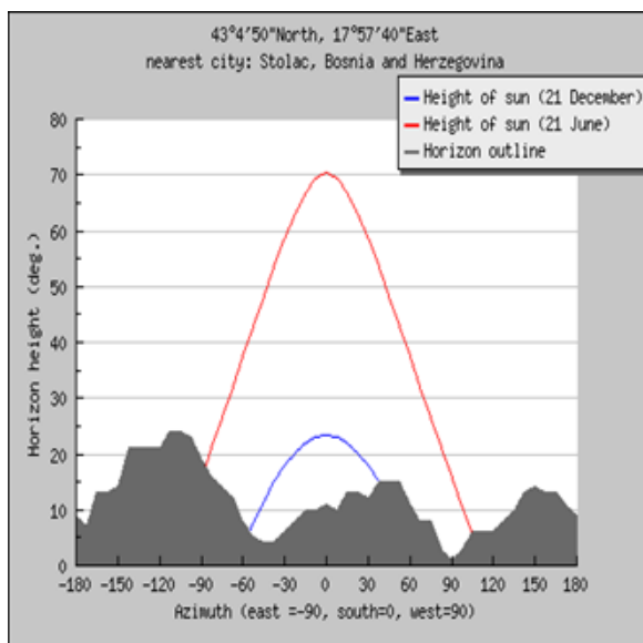
Slika 5.1. Cilindrični Sunčev dijagram [6]
