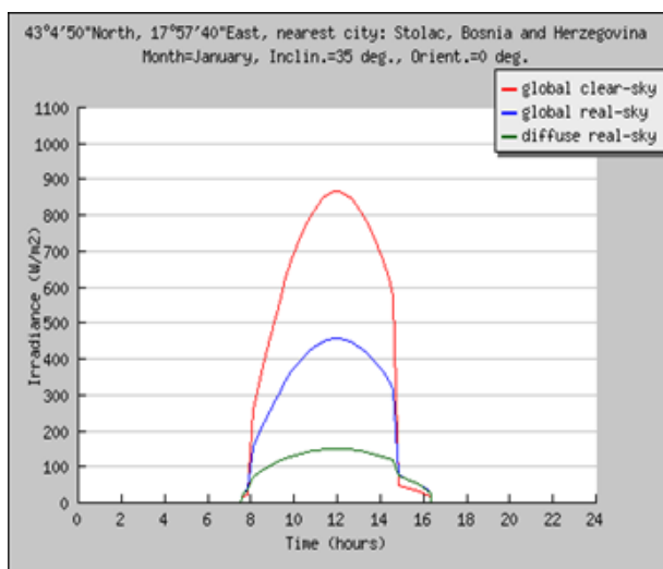
Slika 5.3. Prosječna globalna ozračenost fiksnog panela pod uglom inklinacije od 350 (mjesec juli i januar) za grad Stolac [6]
