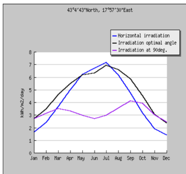
Slika 5.2. Graf Suncevog zračenja za različite plove [6]
